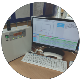
АУ ЦАСПИ ППО с телефонной трубкой и монитором
